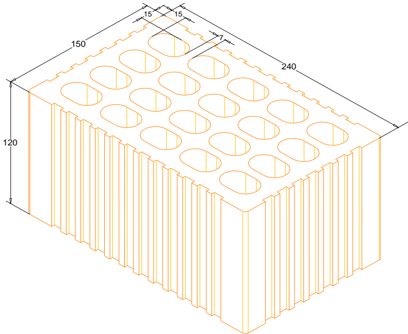
Cotas mm Medidas Nominales
