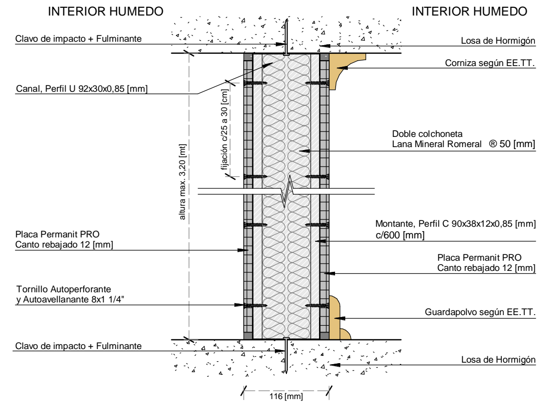
CORTE A-A'
