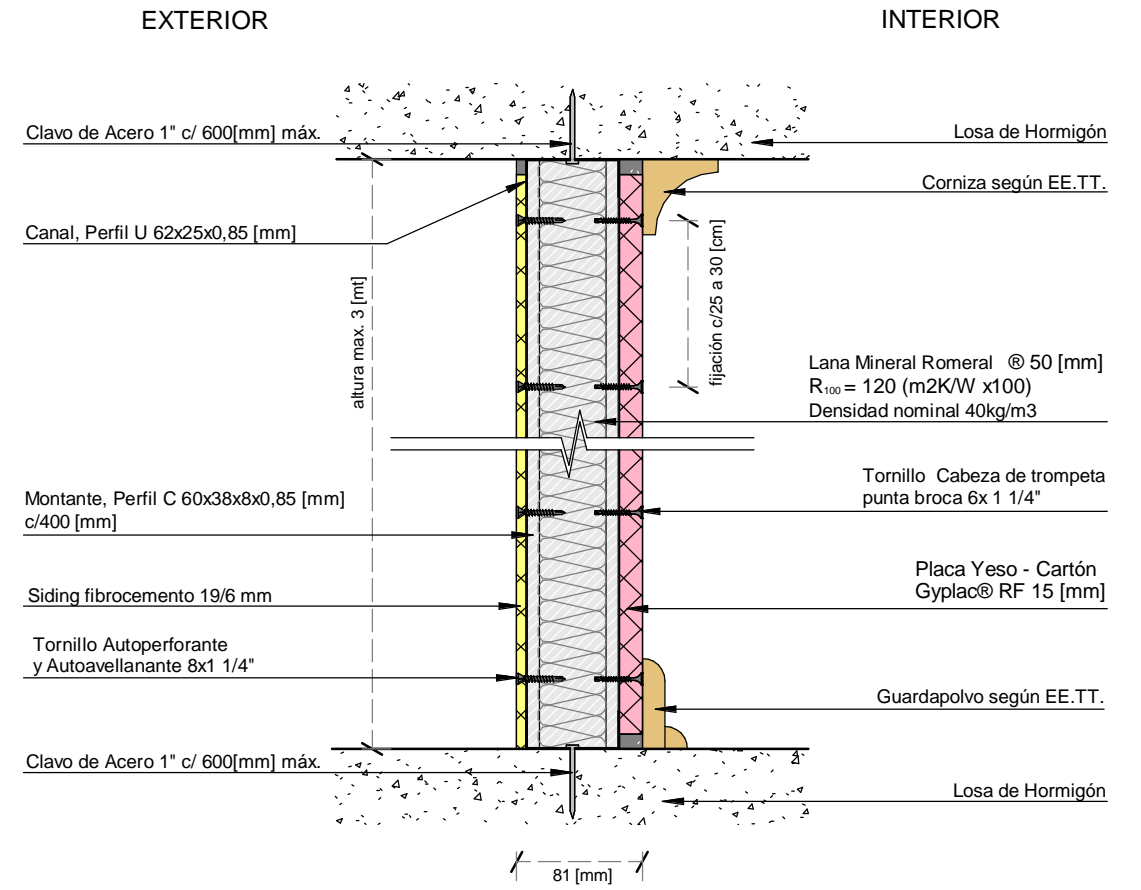
CORTE A-A'
