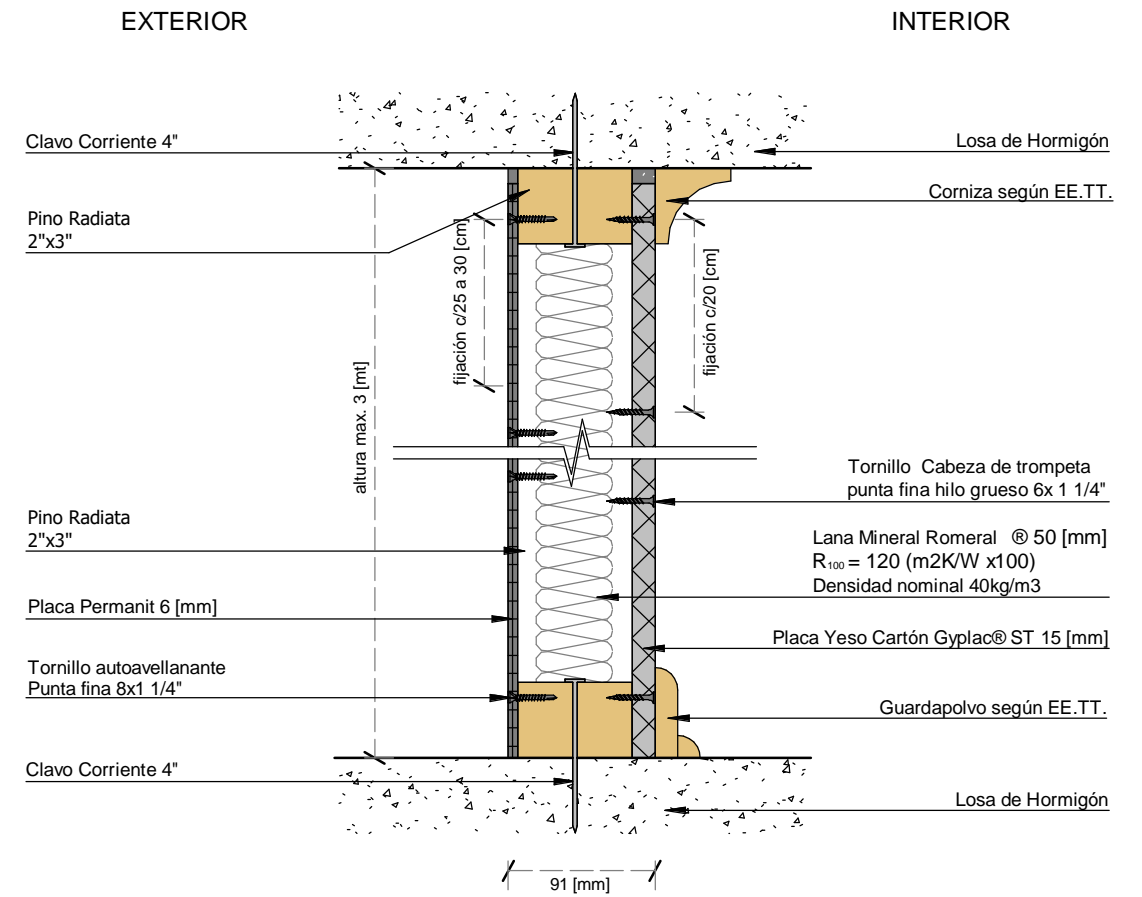
CORTE A-A'
