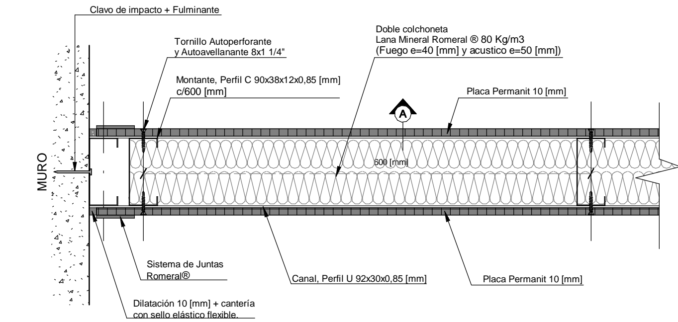
PLANTA
