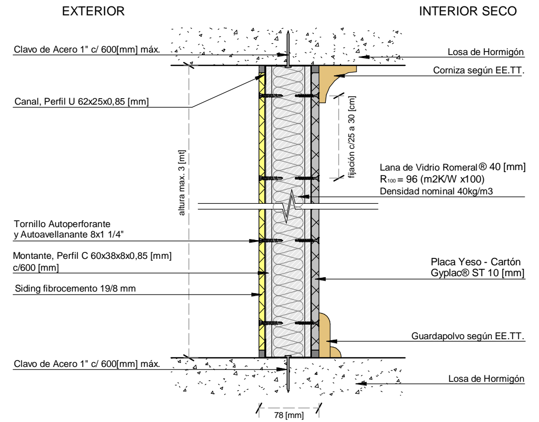
CORTE A-A'
