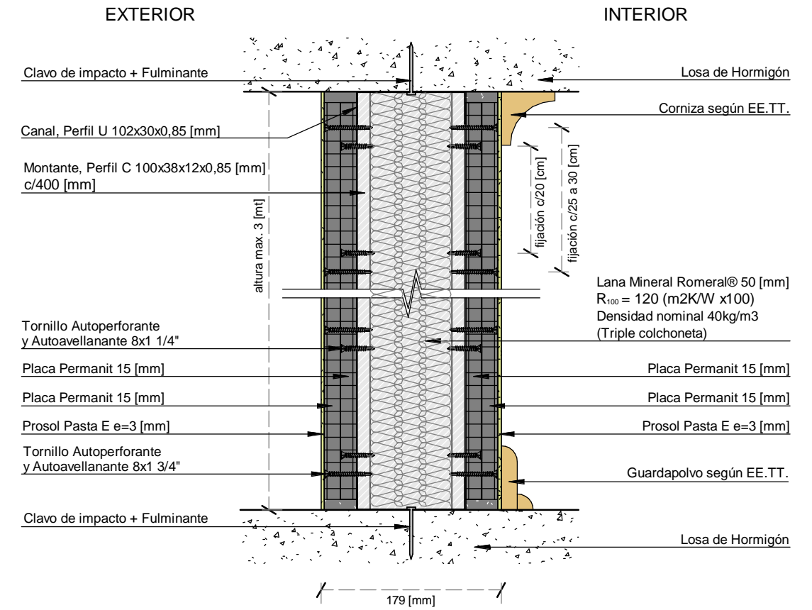
CORTE A-A'
