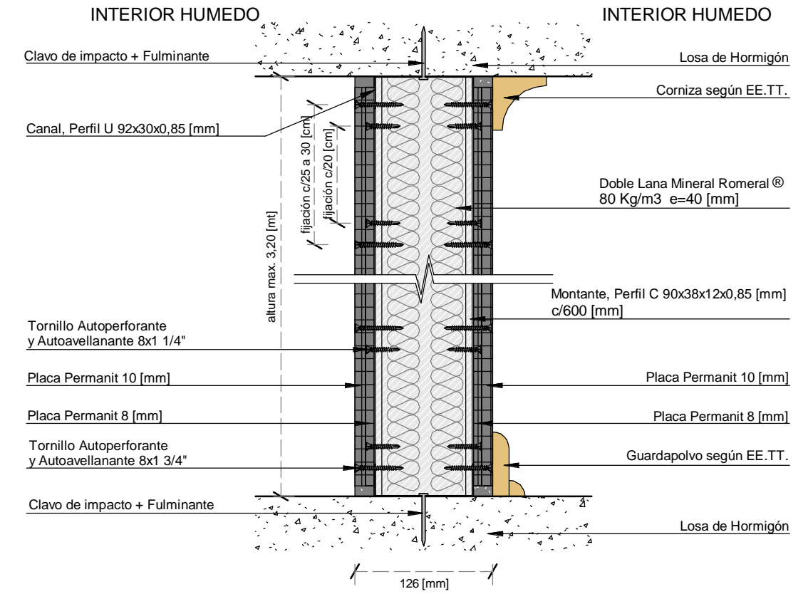
CORTE A-A'
