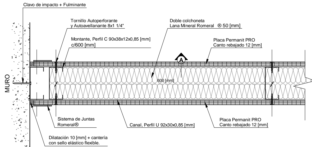
PLANTA
