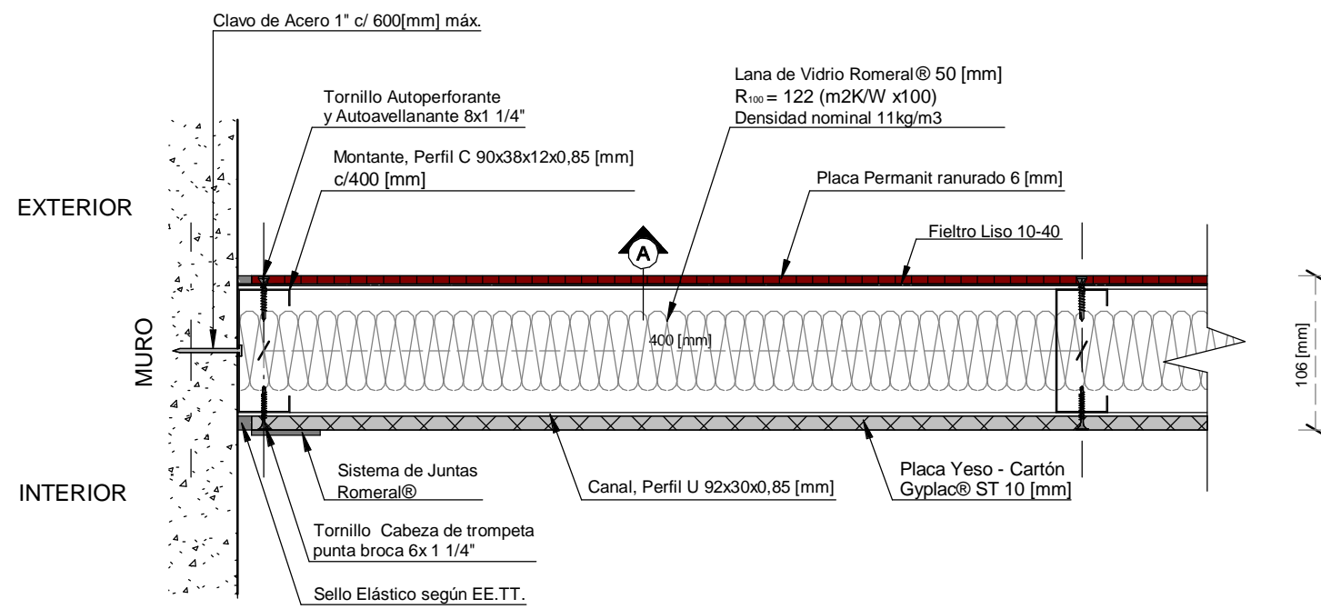
PLANTA
