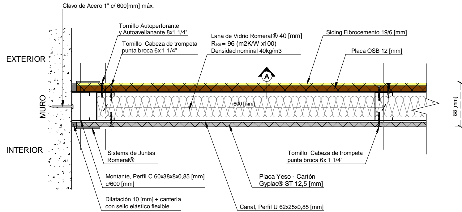
PLANTA
