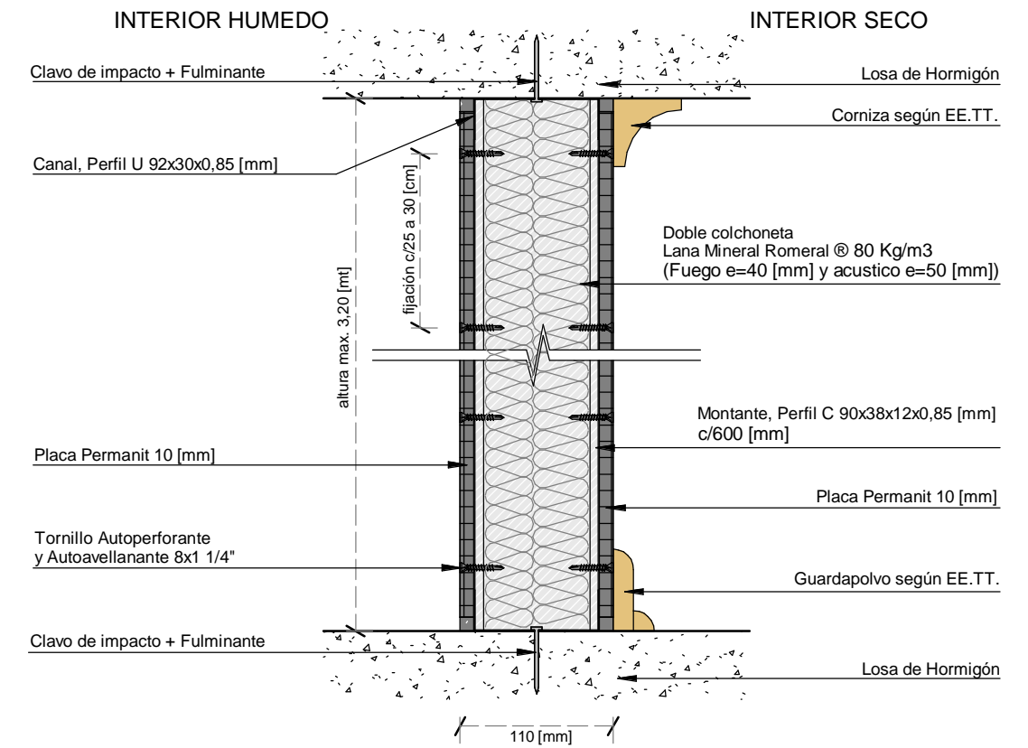
CORTE A-A'
