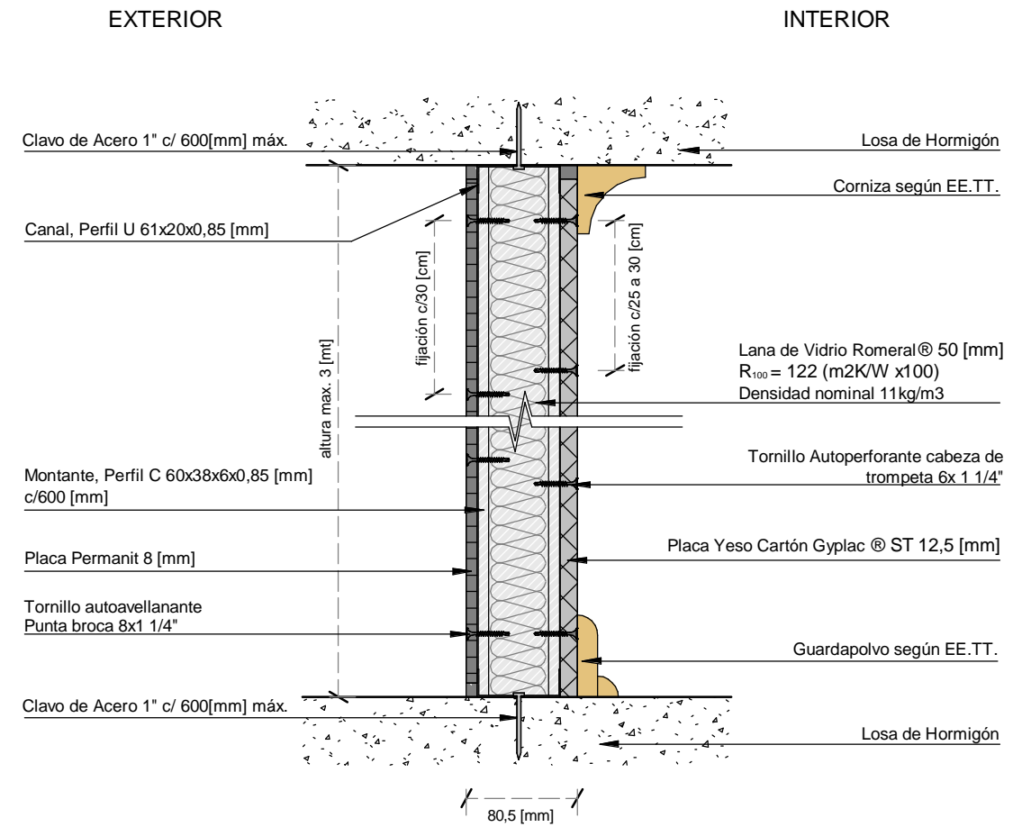
CORTE A-A'
