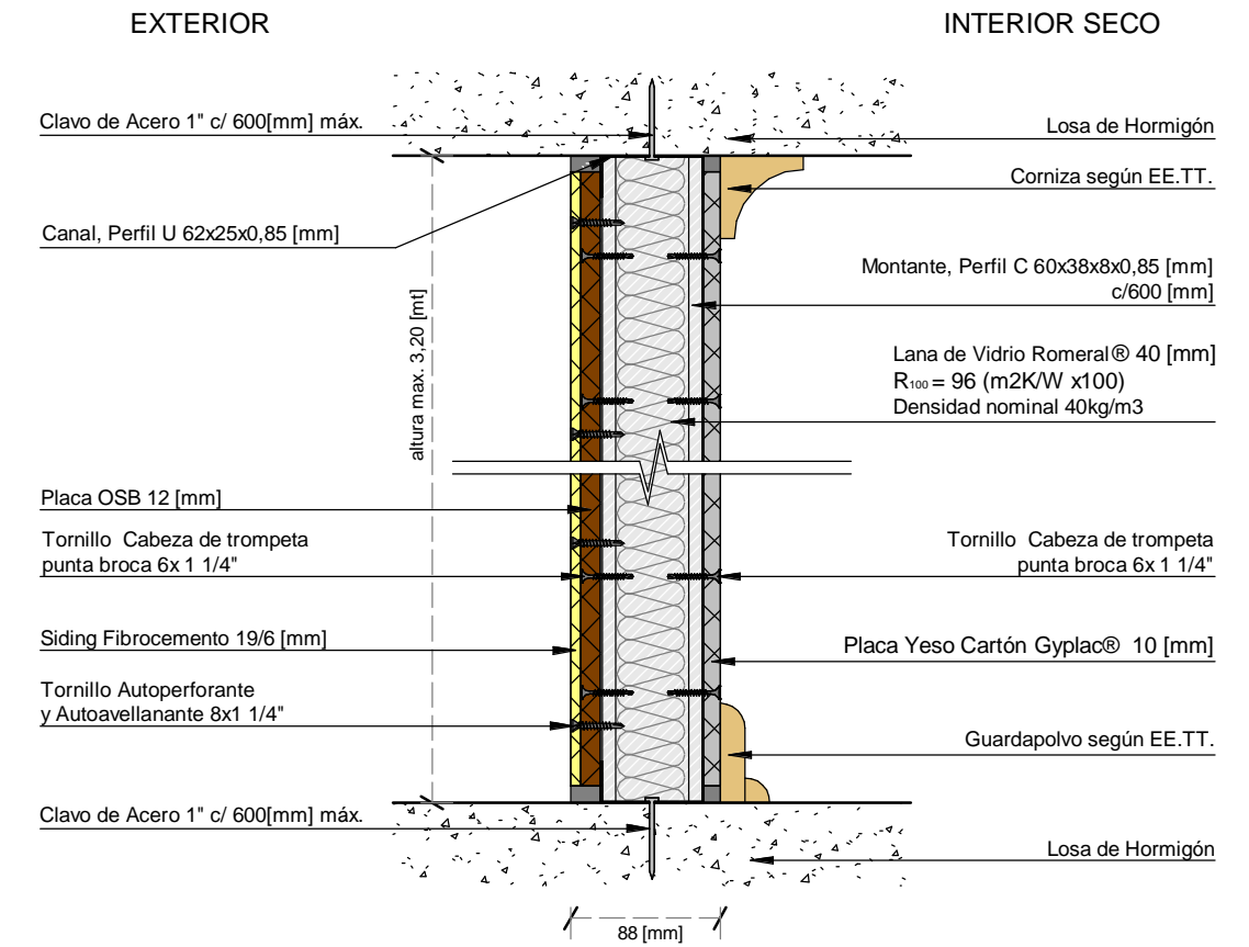
CORTE A-A'
