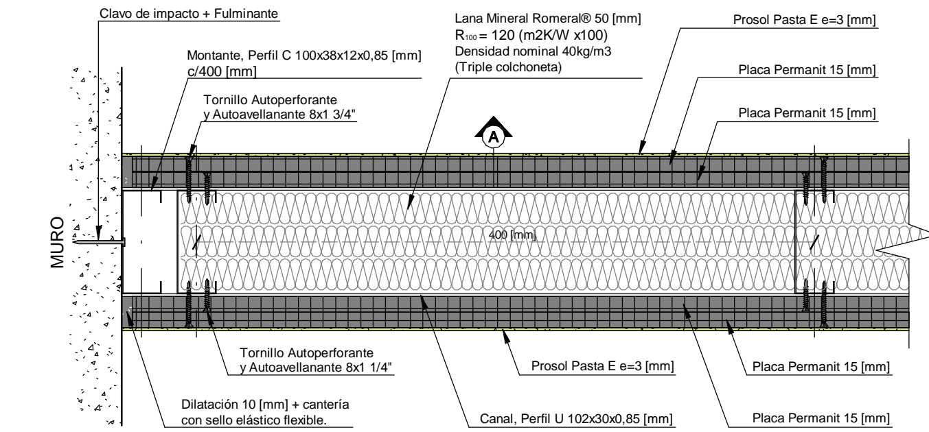
PLANTA
