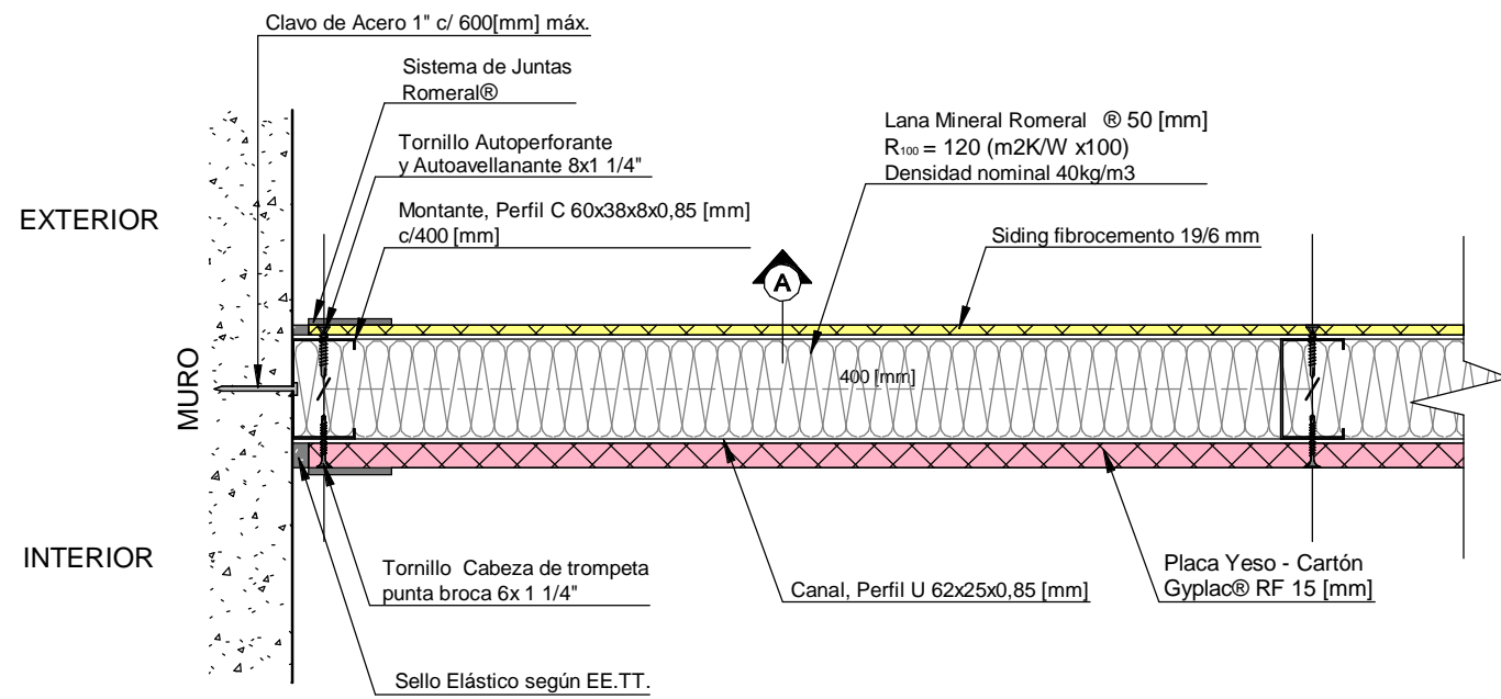
PLANTA
