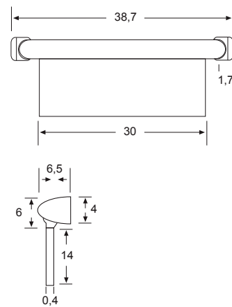
Dimensiones (mm)
