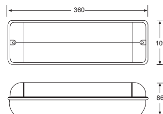
Dimensiones (mm)
