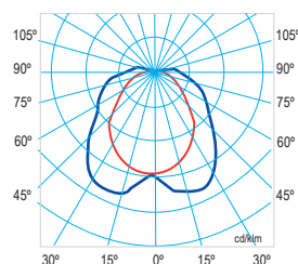
Curva Fotométrica
