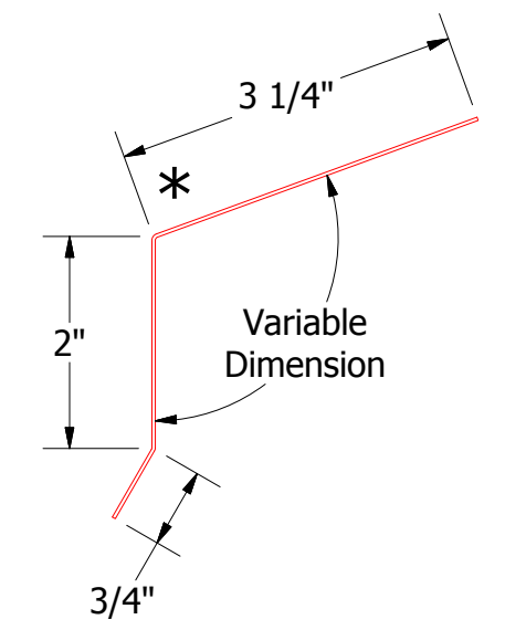
SCA175-Drip Edge
