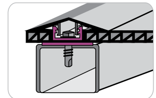
FIJACIÓN EN EL CENTRO
